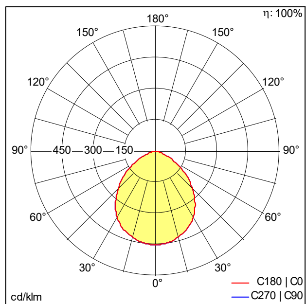
TE_AMY_150_LED_DL_1000_830.ltd
