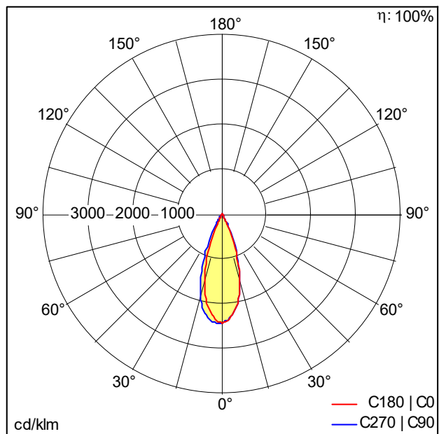
TE_LILY_LED_SPOT_IP44_38_68_600_927.ltd
